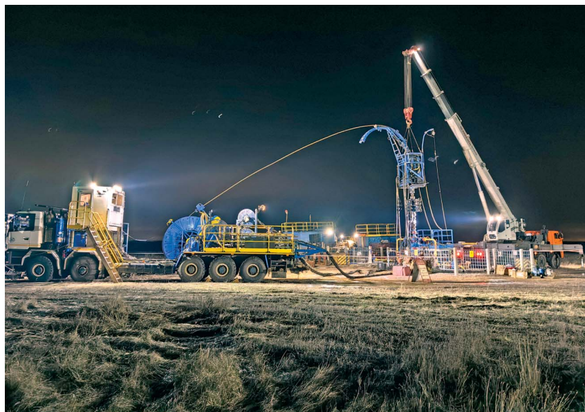
Процесс спуска концентрической лифтовой колонны с применением колтюбинговой установки
