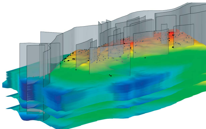
Структурно-тектоническая модель Западного участка Оренбургского НГКМ
